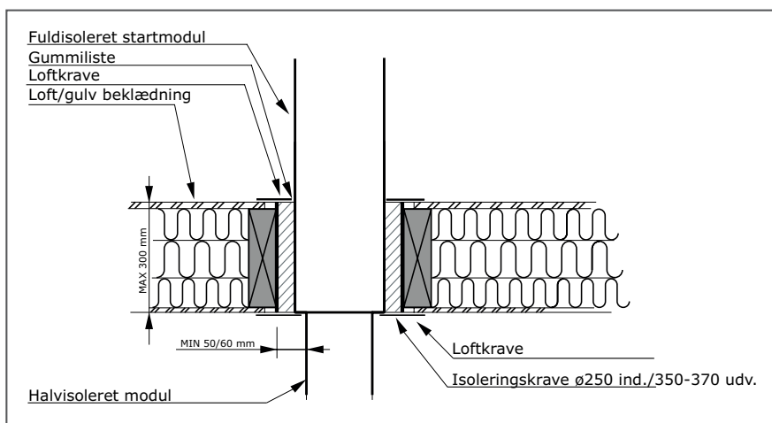
FIG. 2 - Gennemføring i loft/etageadskillelse med skjult overgang
