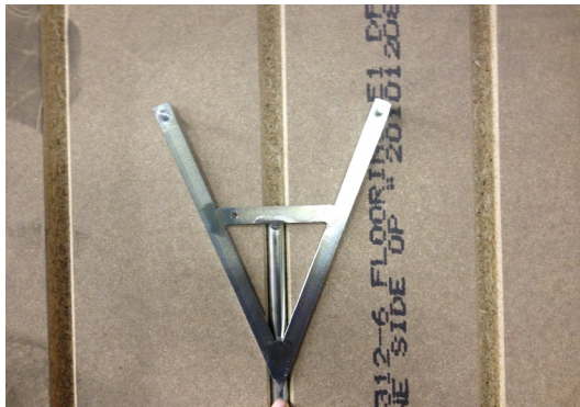
Skabelon delen udlægges i enden af spånpladens spor.
