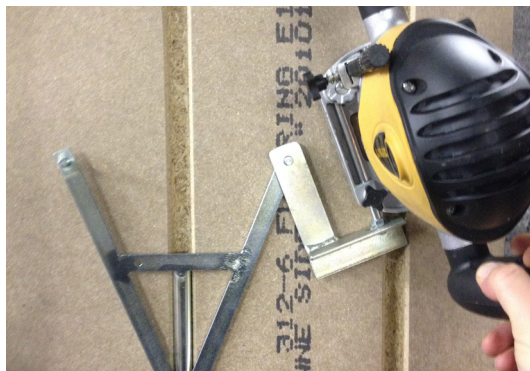
Overfræseren påmonteres ovenpå fræsestyret og skabelonland.
