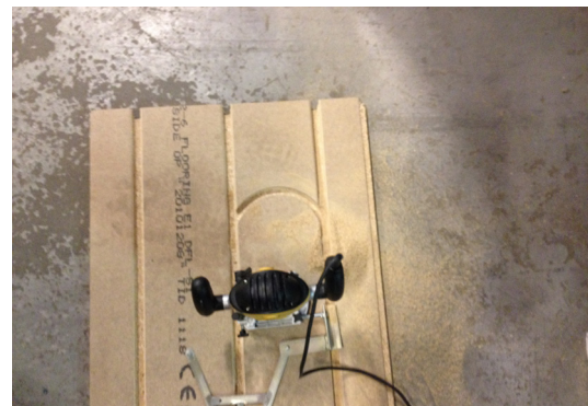
Med overfræseren fræses vendespor i den ønskede dimension.
