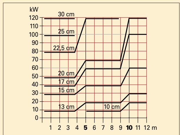
Dimensionering af oliefyrsskorstene.
