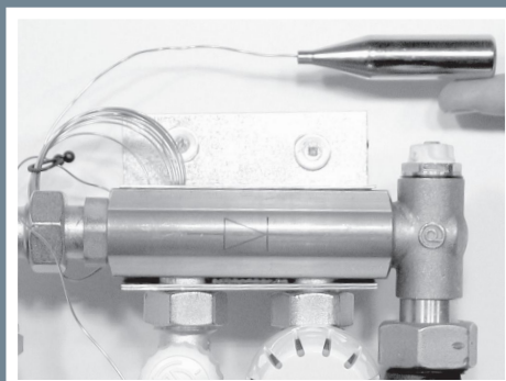
Kapilarrørsføleren placeres i rummet, hvor temperaturen ønskes reguleret
