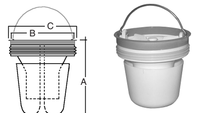
FlexNEPTUN ® med adapter-ring. Passer til ovenstående afløbsskåle
