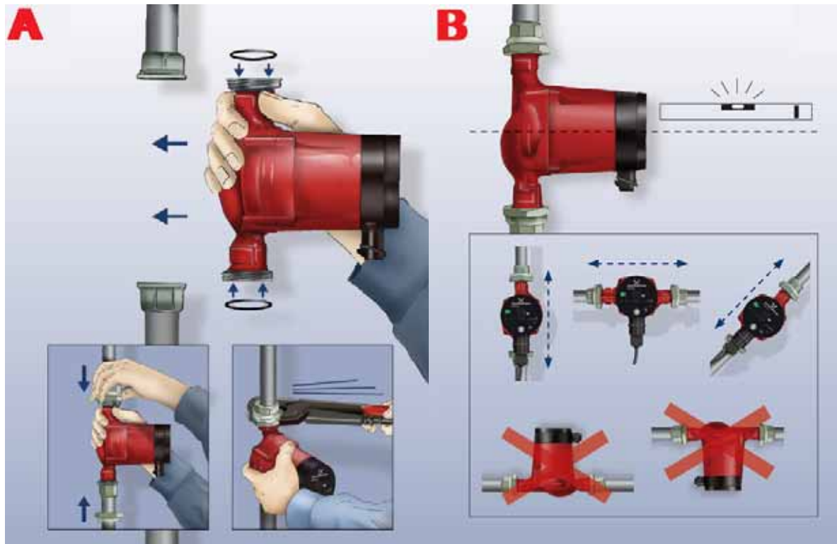
Fig. 3 Montering af GRUNDFOS ALPHA2
