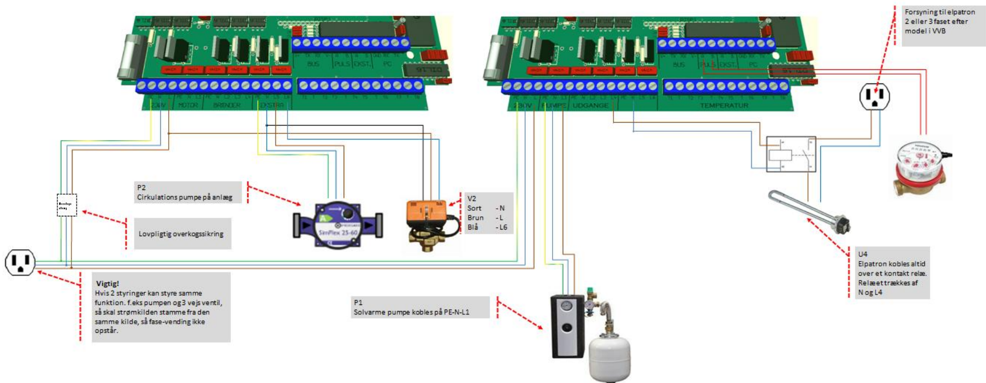
PILLEFYR STYRING
